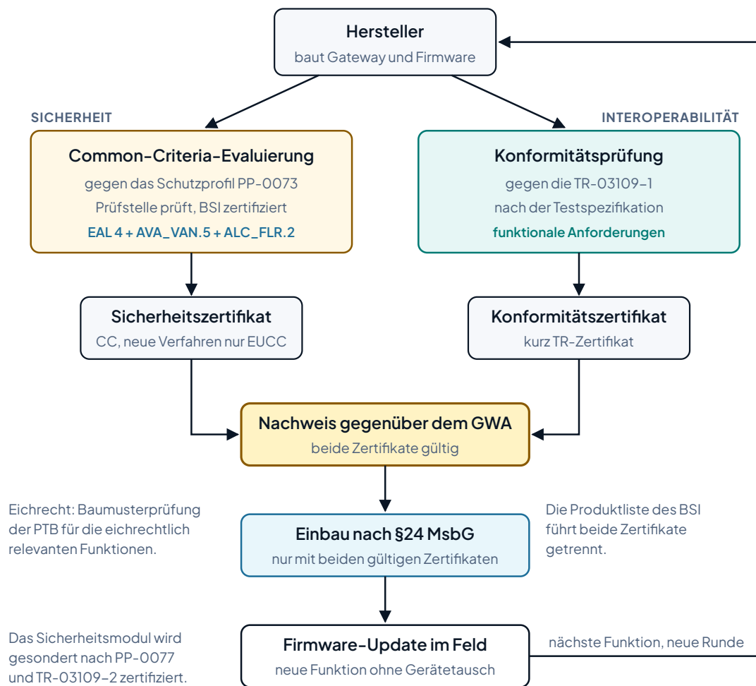
Abbildung 1: Zwei Prüfungen, ein Einbau. Das Gateway braucht ein Sicherheitszertifikat gegen das Schutzprofil PP-0073, neue Verfahren seit dem 27. Februar 2026 nur noch nach EUCC, während bestehende CC-Zertifikate weiter gepflegt werden, und ein Konformitätszertifikat gegen die TR-03109-1, in der Produktliste des BSI kurz TR-Zertifikat. Erst beide zusammen, dem Gateway-Administrator nachgewiesen, erlauben den Einbau. Für die eichrechtlich relevanten Funktionen kommt die Baumusterprüfung der PTB hinzu, und jede neue Funktion beginnt den Kreislauf von vorn.
