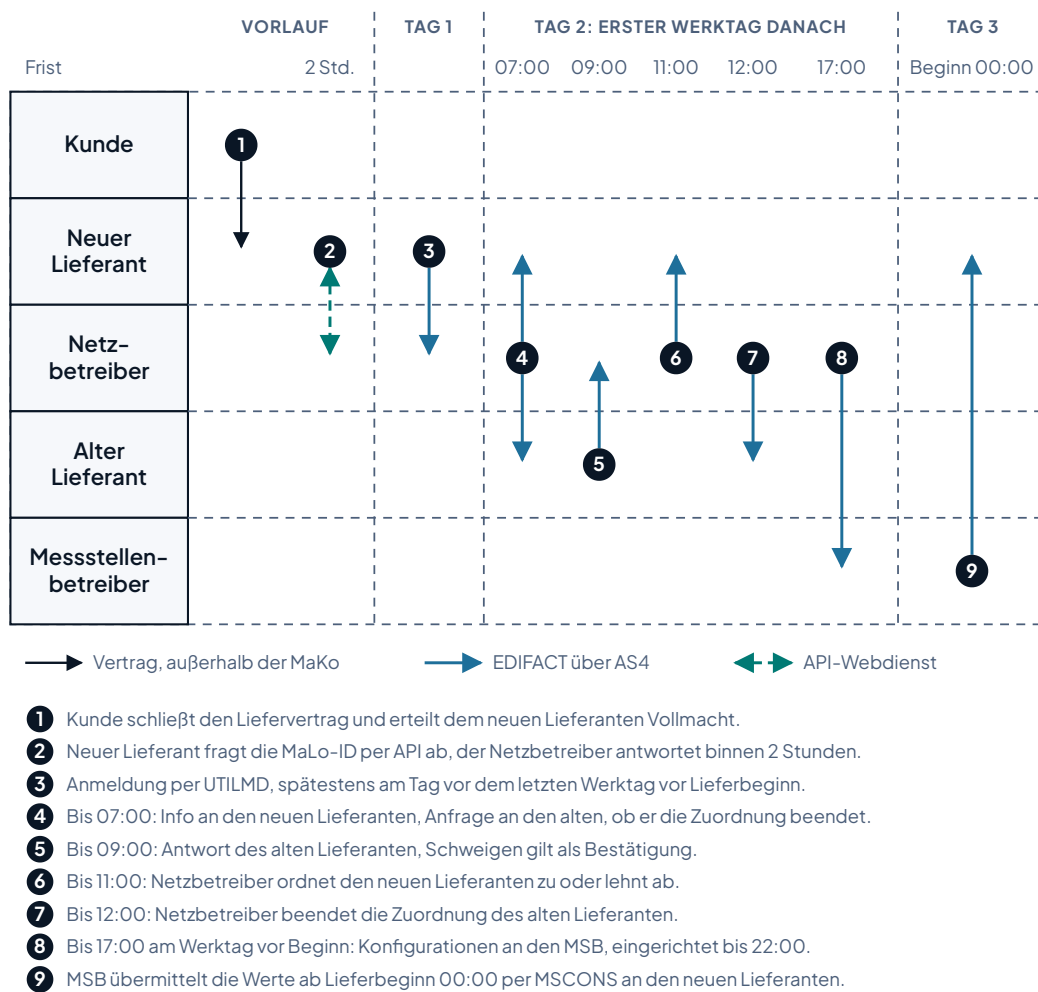
Abbildung 2: Vereinfachte Ablaufdarstellung nach GPKE, keine BPMN-Notation, für eine verbrauchende Marktlotation mit frühestmöglichem Lieferbeginn. Seit dem 1. Januar 2026 muss der technische Vorgang des Wechsels nach §20a EnWG binnen 24 Stunden vollzogen sein, die Fristen aus GPKE Teil 2 und 3 setzen das um. Tag 2 ist der erste Werktag nach der Anmeldung. Dargestellt ist der Fall, dass der alte Lieferant zum Lieferbeginn noch zugeordnet ist. Die empfohlene Kündigung zwischen den Lieferanten vorab fehlt; hat sich der alte Lieferant danach schon abgemeldet, entfallen die Schritte 4, 5 und 7.
