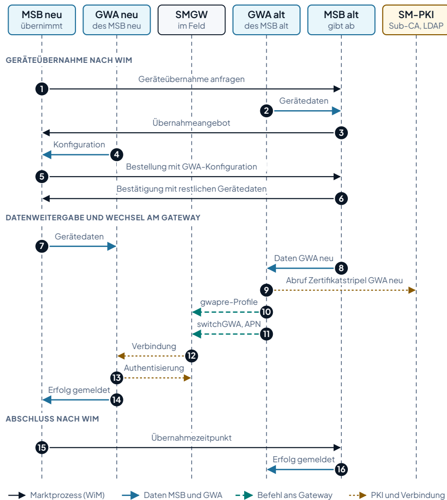
Abbildung 2: Der GWA-Wechsel beim Wechsel des Messstellenbetreibers mit Geräteübernahme nach WiM Strom, vereinfacht nach dem VDE-FNN-Hinweis vom Oktober 2024. Zusammengehörige Schritte sind teils zu einem Pfeil zusammengefasst, die Bahn der SM-PKI ist ergänzt. Die Vorbereitung im Bereich gwapre (Schritt 10) und die Authentisierung als Abschluss (Schritt 13) folgen der TR-03109-1 und ihrer Anlage VI. Wie die Vorlage zeigt die Abbildung nur den Erfolgsfall und nicht den Wechsel allein des Dienstleisters für die Gateway-Administration.
