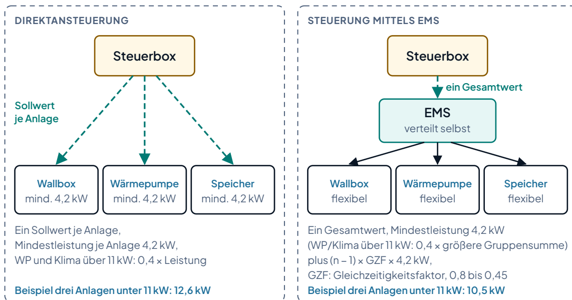
Abbildung 2: Direktansteuerung und Steuerung mittels EMS im Vergleich. Links erhält jede Anlage einen eigenen Sollwert aus der Steuerbox (gestrichelt). Rechts erhält das EMS einen Gesamtwert (gestrichelt) und verteilt ihn nach Vorgabe des Betreibers auf die Anlagen (durchgezogen). Beide Beispiele rechnen mit drei Anlagen unter 11 kW.
