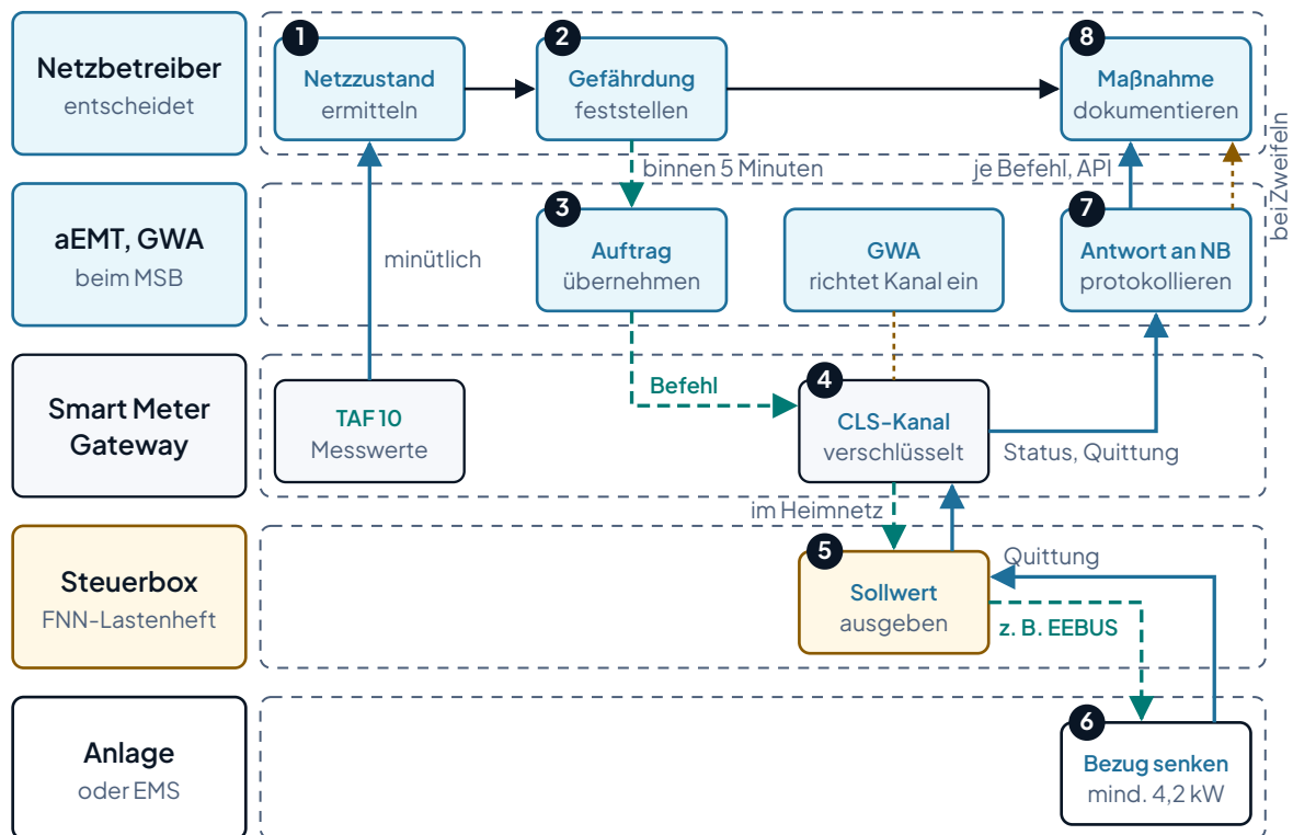
Abbildung 1: Vereinfachte Ablaufdarstellung, keine BPMN-Notation. Die nummerierten Schritte führen von der Netzzustandsermittlung über den Steuerbefehl zur Antwort, die der Messstellenbetreiber zu jedem Befehl an den Netzbetreiber schickt, und zur Dokumentation beim Netzbetreiber. Gestrichelt: Steuerbefehl; durchgezogen blau: Messwerte, Quittung und Antwort; durchgezogen in Schriftfarbe: Ablauf beim Netzbetreiber; gepunktet: Einrichtung des CLS-Kanals durch den Gateway-Administrator und Abruf der Protokolle bei Zweifeln. Minütliche TAF-10-Werte sind eine Zusatzleistung nach §34 MsbG.
