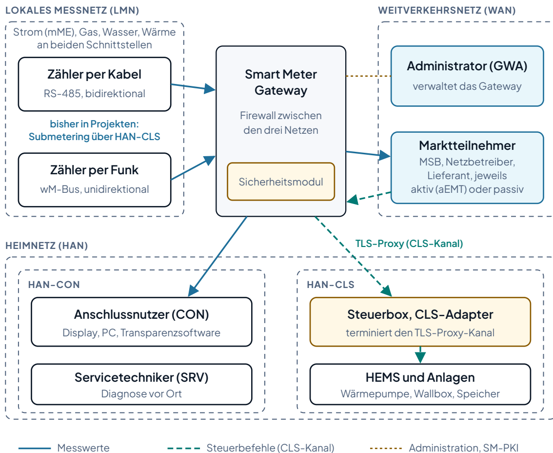
Abbildung 2: Die drei Netze des Smart Meter Gateway. Zähler liefern über das LMN, Submetering kommt in den öffentlich beschriebenen Projekten über einen Adapter im HAN-CLS. Das Gateway schickt Messwerte an die Marktteilnehmer im WAN und an den Kunden im HAN. Der Gateway-Administrator verwaltet das Gerät über die Smart-Metering-PKI. Steuerbefehle schickt nur ein aktiver externer Marktteilnehmer, sie laufen durch den TLS-Proxy des Gateway zur Steuerbox im HAN-CLS.
