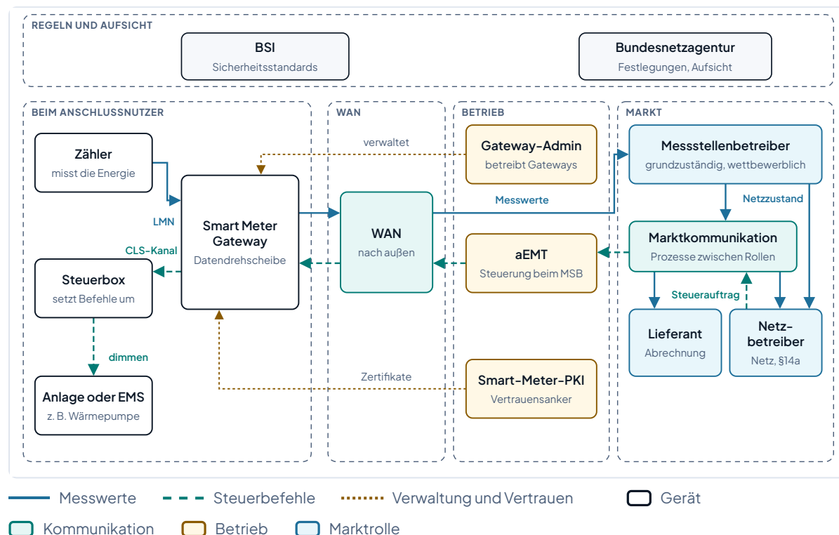
Abbildung: Das Modell in der fachlichen Sicht. Durchgezogene Linien sind Messwerte, gestrichelte Steuerbefehle, gepunktete Verwaltung und Vertrauen. Die Schnittstellen dahinter nennt die Textfassung je Knoten unter „Technisch“.
