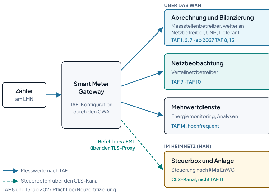
Abbildung 1: Wohin die Tarifierungsfälle liefern. Abrechnung und Bilanzierung, Netzbeobachtung und Mehrwertdienste laufen über TAF. Abrechnungswerte gehen an den Messstellenbetreiber, der sie nach §60 MsbG an Netzbetreiber, Übertragungsnetzbetreiber und Lieferant weitergibt. Viertelstündliche Netzzustandsdaten nach TAF 10 sind Standard, minutliche eine Zusatzleistung. Die Steuerung nach §14a läuft über den CLS-Kanal zur Steuerbox, nicht über TAF 11. Den Befehl schickt ein aktiver externer Marktteilnehmer.
