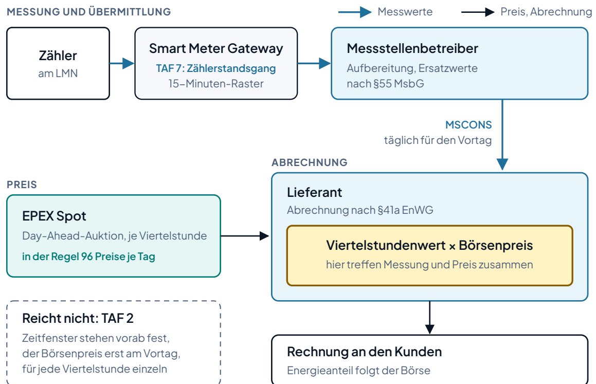
Abbildung 1: Wo Viertelstunde und Preis zusammenkommen. Das Gateway erfasst in der Regel über TAF 7 den Zählerstandsgang, der Messstellenbetreiber schickt ihn täglich im Format MSCONS an den Lieferanten. Aus der Day-Ahead-Auktion kommen in der Regel 96 Preise je Tag. Verrechnet werden beide Reihen erst in der Abrechnung des Lieferanten. Das Netzentgelt, mit Modul 3 ebenfalls zeitvariabel, ist nicht dargestellt.
